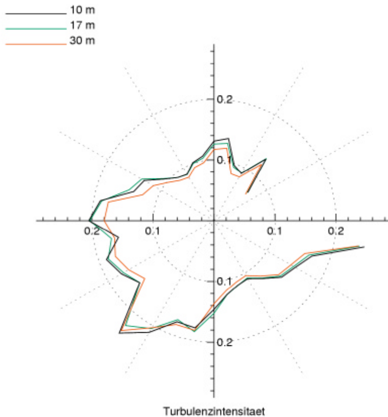
Abb 16. Turbulenzrose am Standort Gotthard in den Höhen 10, 17 und 30 m.
