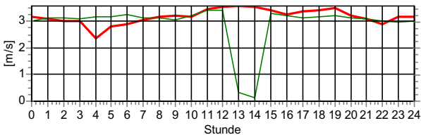
— Windgeschwindigkeit. Höhe: 10.0 m — Windrichtung. Höhe: 10.0 m
