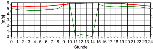
— Windgeschwindigkeit. Höhe: 30.0 m — Windrichtung. Höhe: 30.0 m
