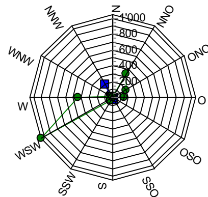
Windenergieerose (kWh/m2/Jahr)
