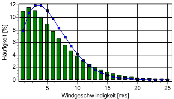
Weibull-Verteilung
