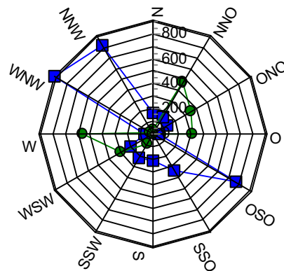
Windenergieerose (kWh/m2/Jahr)
