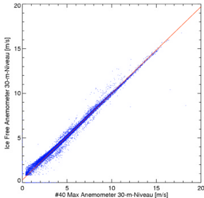
Abb 6. Korrelation der Messungen des Ice Free Anemometers mit den Messungen des #40 Max Anemometers auf 30 m. Die Gleichung der Regressionsgerade gilt für Werte ab 3 m/s: y = 0.970x + 0.308 .
